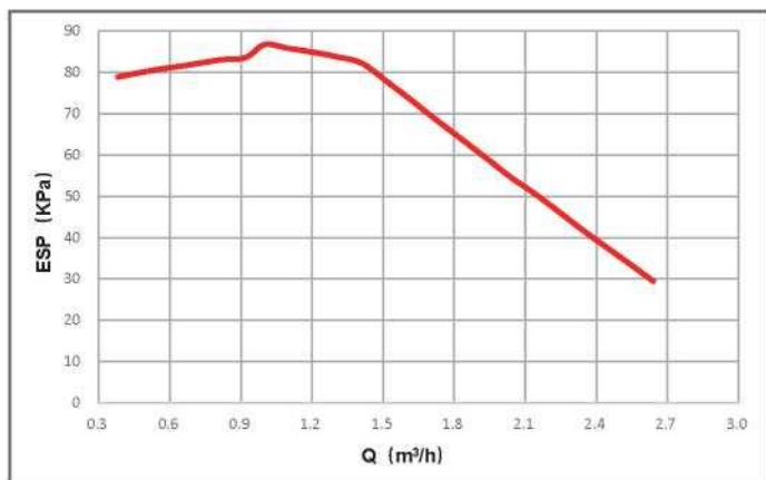
Vnútročná jednotka 60, 100
